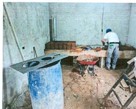
Foto 4: Instalación de elementos faltantes en el área de cocina
